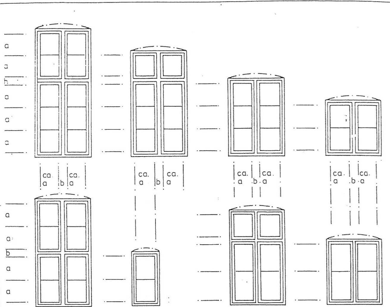
Proportionen und Teilung der Fenster bei Außenwandflächen aus Fachwerk oder Ziegelsichtmauerwerk
