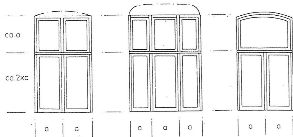
Proportionen und Teilung der Fenster bei Außenwandflächen aus Ziegelsichtmauerwerk oder Putz
